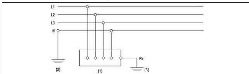
Figuur 3.4. TT-net
