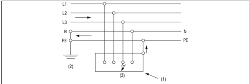
Figuur 4.3. Foutlus in een TN-S-systeem
