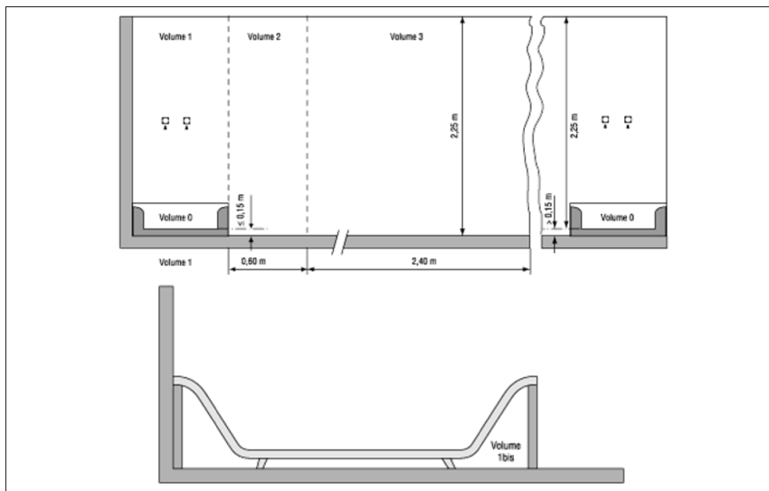
Figuur 7.11. Stortbadkuip — Vooraanzicht
