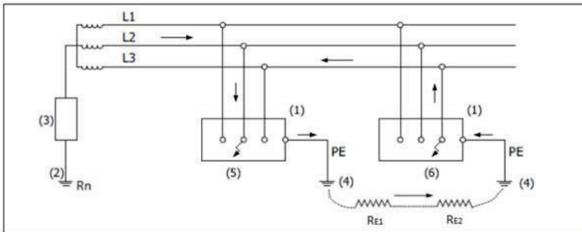
Figuur 4.9. IT-net (twee fouten met niet-verbonden massa's)
