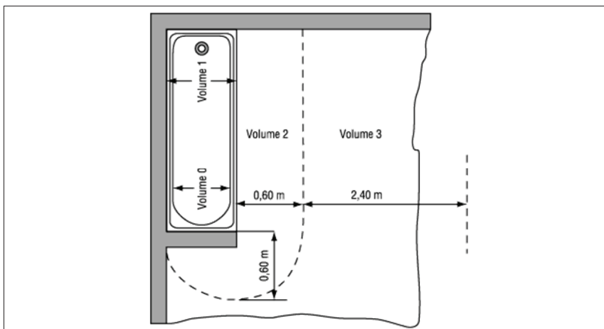
Figuur 7.2. Badkuip met vaste wand
