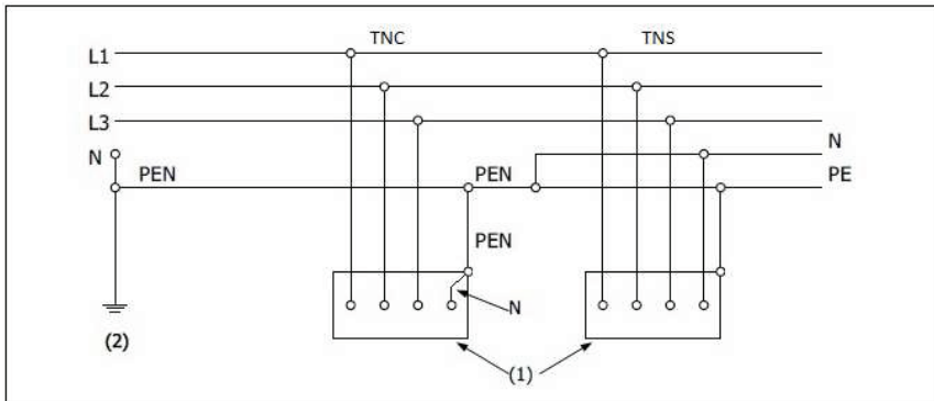
Figuur 2.3. TN-C-S-systeem
