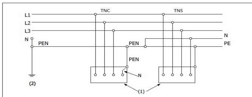
Figuur 3.3. TN-C-S-net
