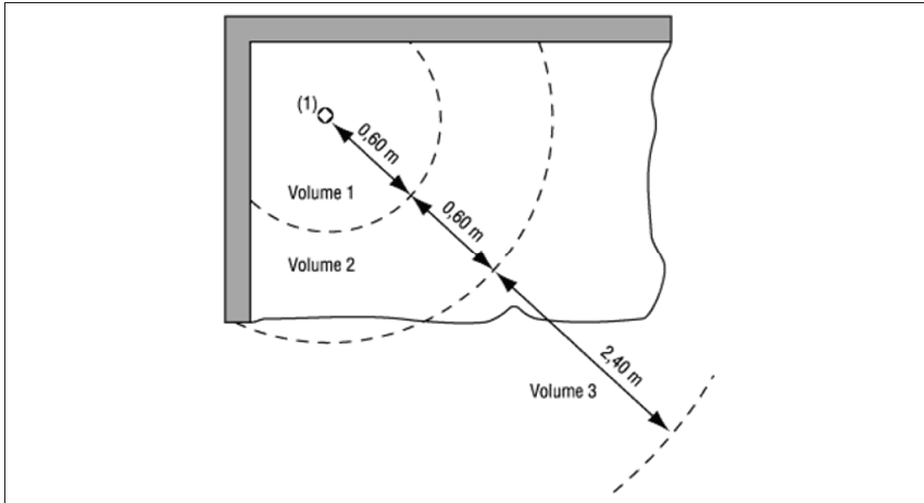
Figuur 7.5. Stortbad zonder kuip
