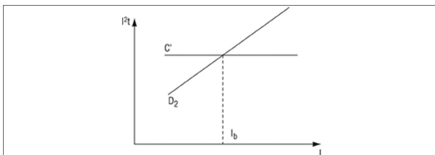
Figuur 5.31. Keuze van de beschermingsinrichting tegen kortsluitingen bij automatische schakelaars (veronderstelde kortsluitstroom)
