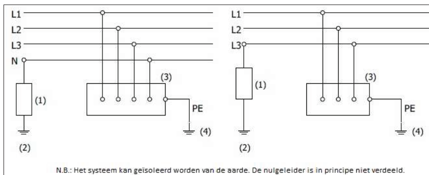
Figuur 2.5. IT-systeem
