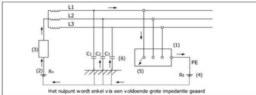
Figuren 4.7. IT-net (Eerste fout)
