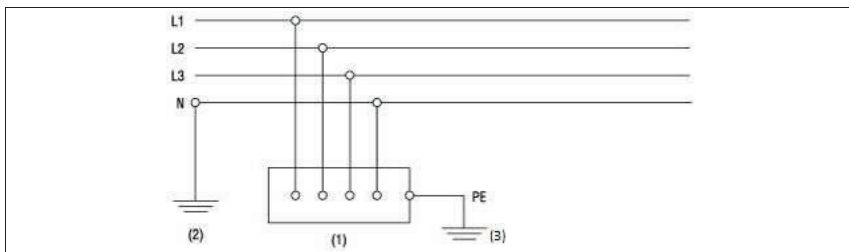
Figuur 2.4. TT-systeem
