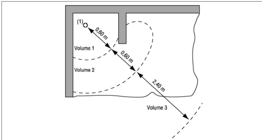
Figuur 7.6. Stortbad zonder kuip, met vaste wand
