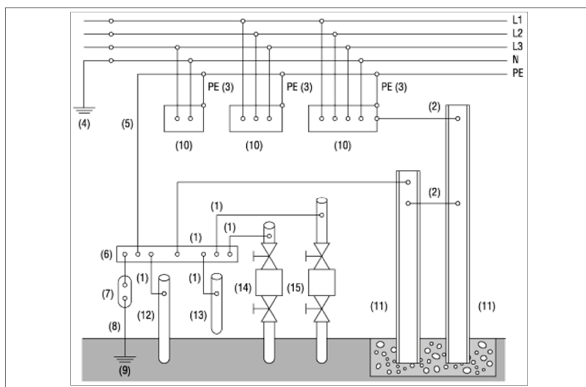
Figuur 2.10. Aardingsinstallatie
