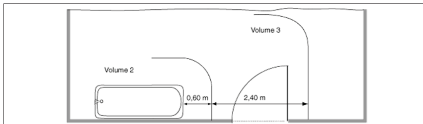
Figuur 7.9. Badkamer: volume 3 begrenst zich tot het binnengedeelte van de badkamer
