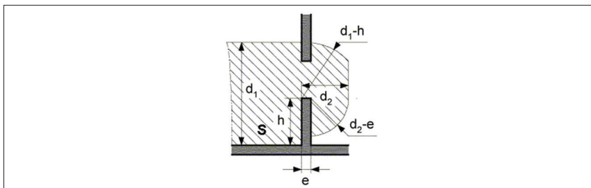
Figuur 2.8. Genaakbaarheidsgabarit: materiële elementen die het verplaatsingsoppervlak begrenzen hebben openingen die geen doorgang verlenen aan een lange staaf van 12 mm diameter
