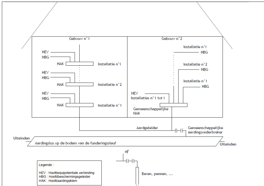
Figuur 5.32. Principeschema van de gemeenschappelijke aardverbinding (Gevalle bedoeld in punt c.1., 1 ste en 2 de alinea)
