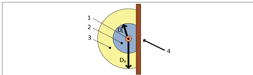
Figuur 2.22. Voorstelling van de zone onder spanning en de nabijheidszone met isolerende bescherminrichting
