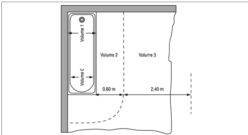
Figuur 7.1. Badkuip
