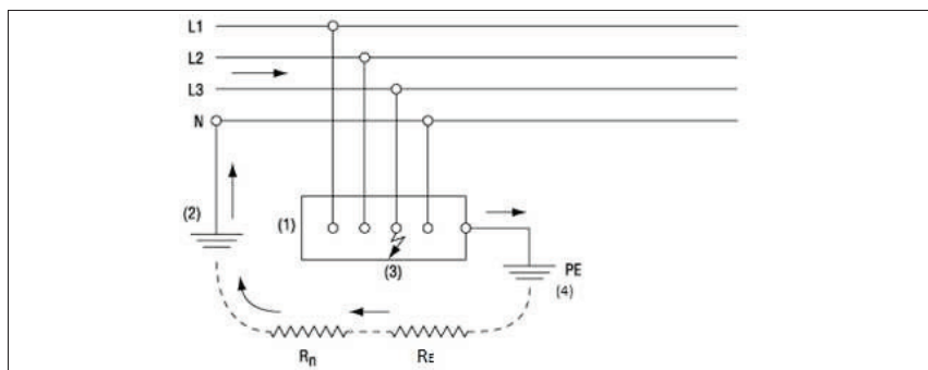
Figuur 4.6. Foutlus in een TT-systeem
