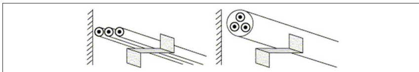
Figuur 5.10. Plaatsingswijzen van elektrische leidingen — Haken
