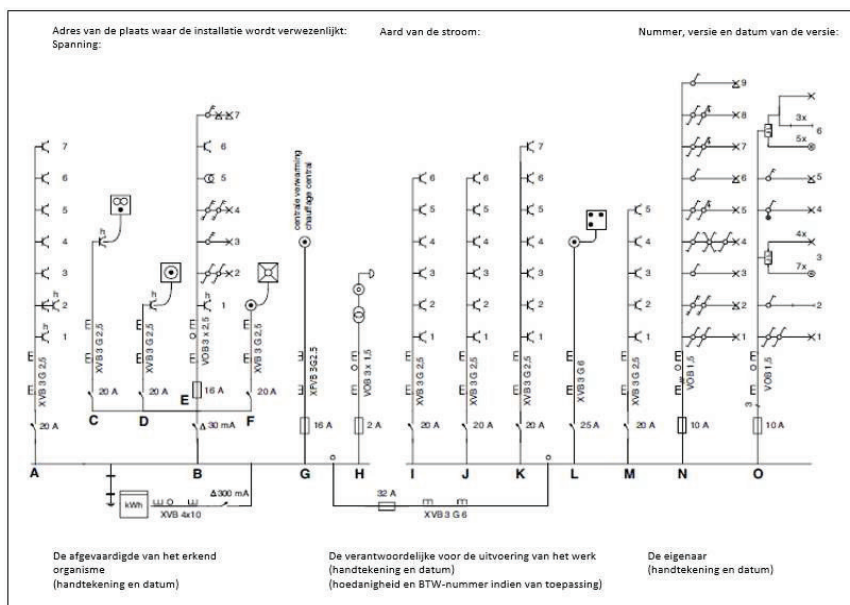
Figuur 3.1. Voorbeeld van een eendraadsschema
