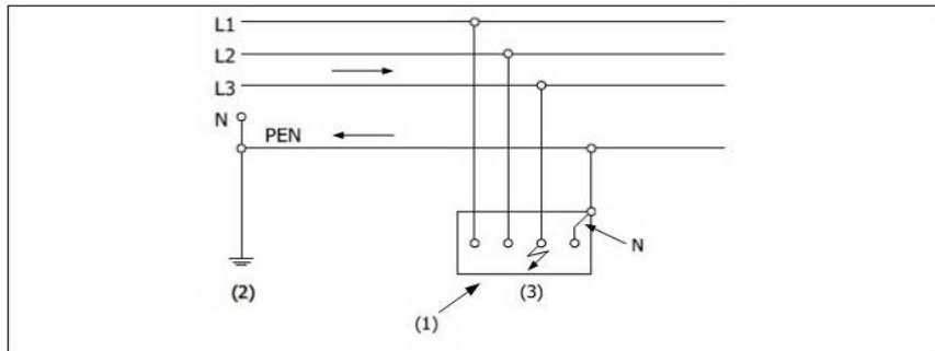
Figuur 4.4. Foutlus in een TN-C-systeem
