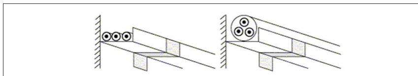
Figuur 5.9. Plaatsingswijzen van elektrische leidingen — Kabelrekken
