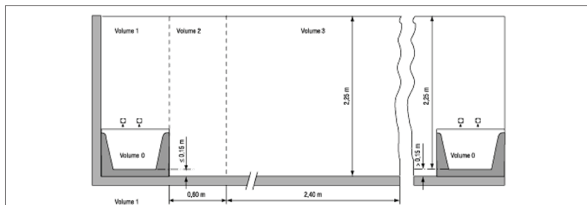
Figuur 7.10. Badkuip — Vooraanzicht
