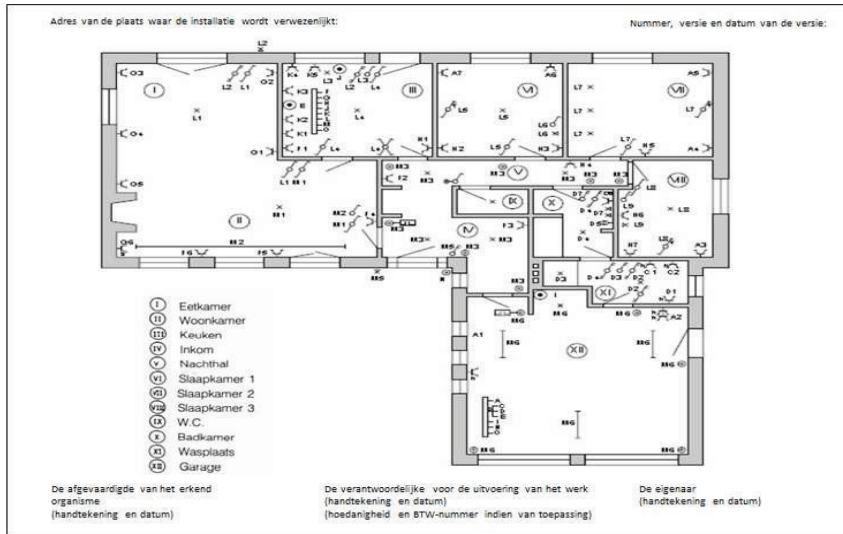
Figuur 3.2. Voorbeeld van een situatieplan
