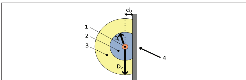
Figuur 2.23. Voorstelling van de zone onder spanning en de nabijheidszone met geaarde, metalen bescherminrichting
