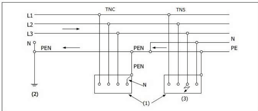
Figuur 4.5. Foutlus in een TN-C-S-systeem
