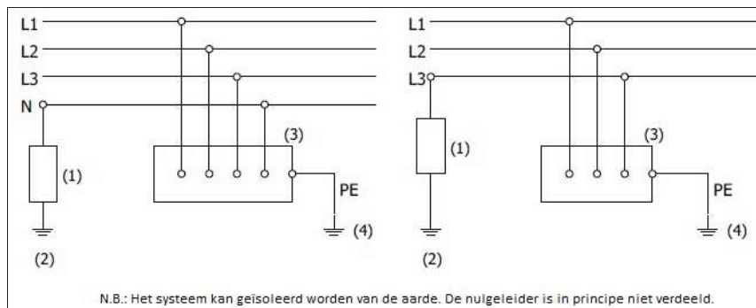
Figuur 3.5. IT-net
