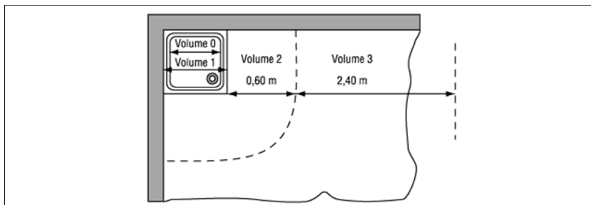
Figuur 7.3. Stortbadkuip
