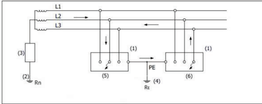
Figuur 4.8. IT-net (twee fouten met verbonden massa's)
