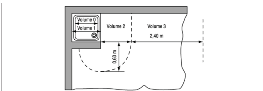
Figuur 7.4. Stortbadkuip met vaste wand
