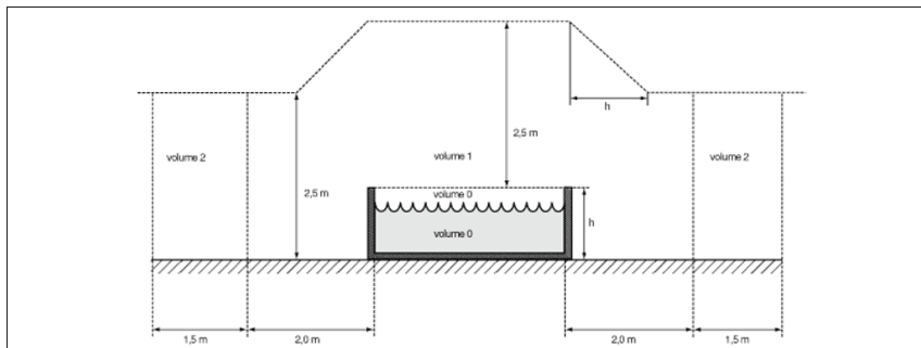
Figuur 7.13. Zwembaden: afmetingen van de volumes voor bovengrondse kommen
