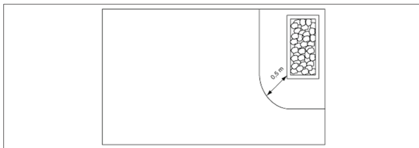
Figuur 7.16. Verschillende volumes van sauna's — Bovenaanzicht
