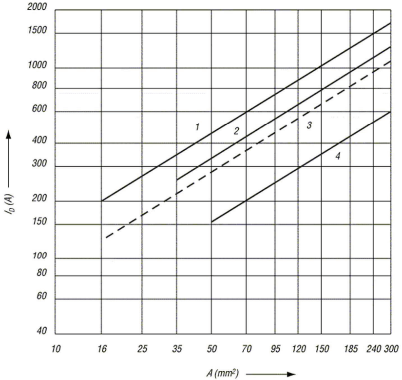
Figuur 5.46. Stroom I_D voor de aardgeleiders met ronde doorsnede in functie van hun doorsnede ( A in \text{mm}^2 )
