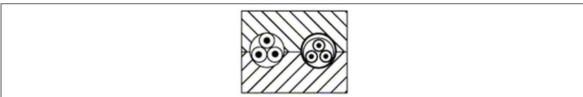
Figuur 5.37. Plaatsingswijzen van elektrische leidingen — Geprefabriceerde blokken
