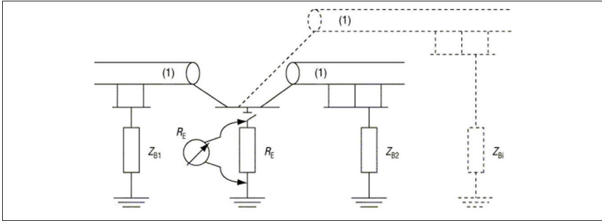
Figuur 2.13. Aardingsweerstand R_E
