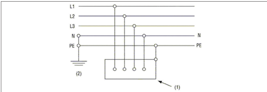
Figuur 2.1. TN-S-systeem
