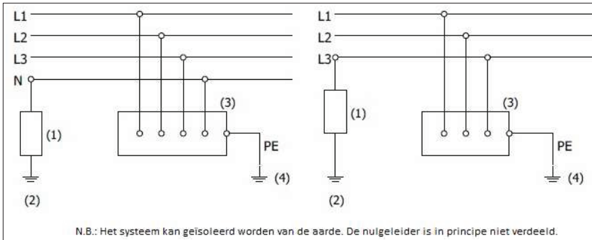
Figuur 3.3. IT-net
