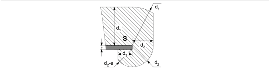
Figuur 2.7. Genaakbaarheidsgabariet: het verplaatsingsoppervlak is begrensd door een materieel element
