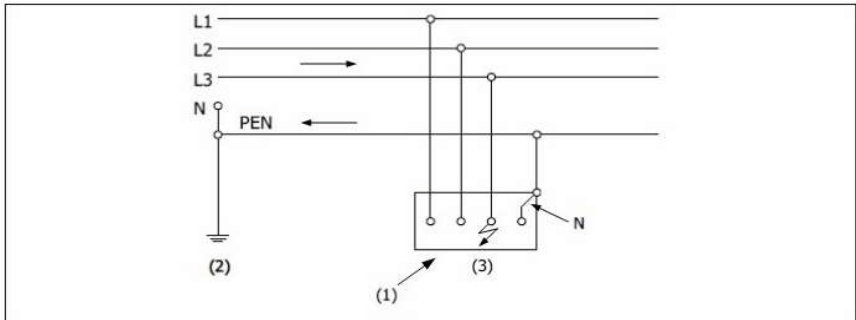
Figuur 4.4. Foutlus in een TN-C-systeem
