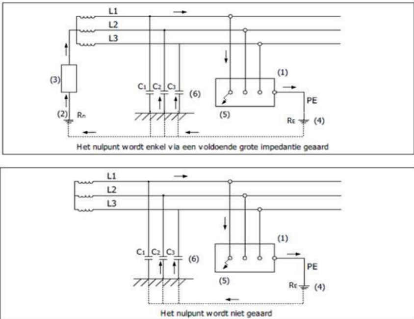
Figuren 4.7. IT-net (Eerste fout)
