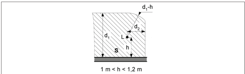
Figuur 2.7. Genaakbaarheidsgabariet: het verplaatsingsoppervlak is begrensd door een materieel element
