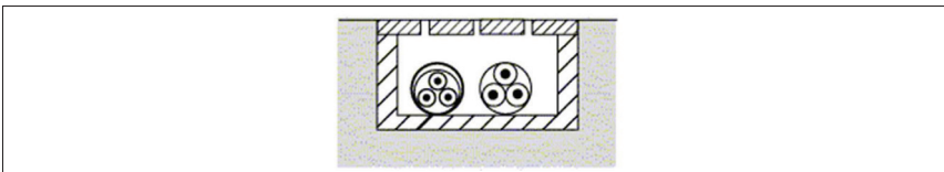
Figuur 5.32. Plaatsingswijzen van elektrische leidingen — Buizen in open of verluchte kabelkanalen
