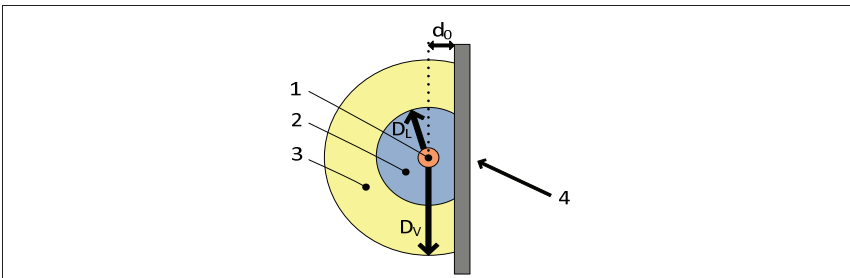
Figuur 2.30. Voorstelling van de zone onder spanning en de nabijheidszone met geaarde, metalen bescherminrichting
