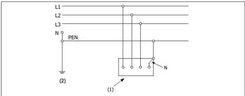
Figuur 2.2. TN-C-systeem
