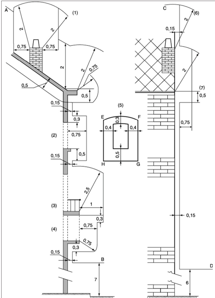
Figuur 7.1. Afstanden ten opzichte van gebouwen
