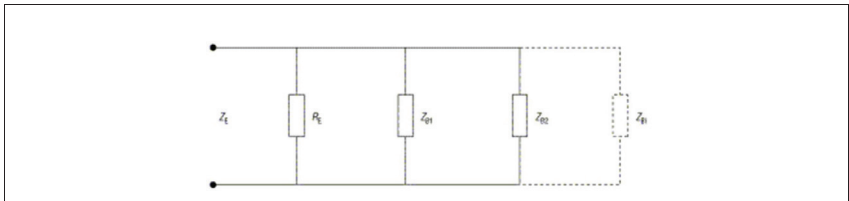
Figuur 2.15. Equivalent schema van de aardingsimpedantie Z_E
