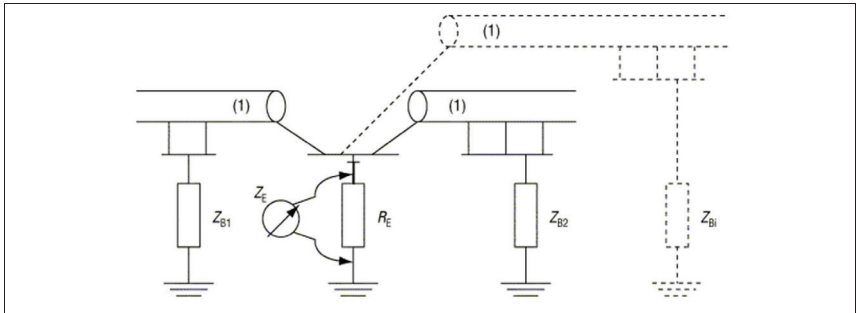
Figuur 2.14. Aardingsimpedantie Z_E
