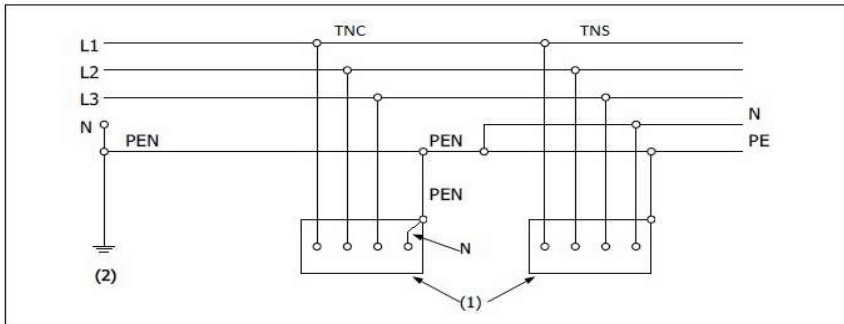
Figuur 3.1. TN-C-S-net
