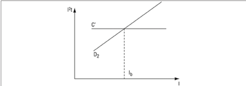
Figuur 5.45. Keuze van de beschermingsinrichting tegen kortsluitingen bij automatische schakelaars (veronderstelde kortsluitstroom)
