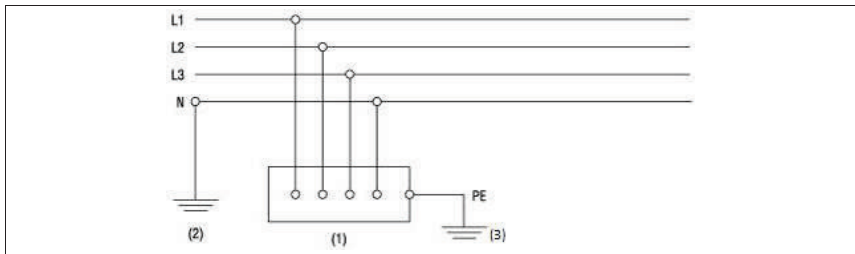
Figuur 3.2. TT-net
