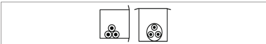
Figuur 2.22. Plaatsingswijze «kabelbaan»
