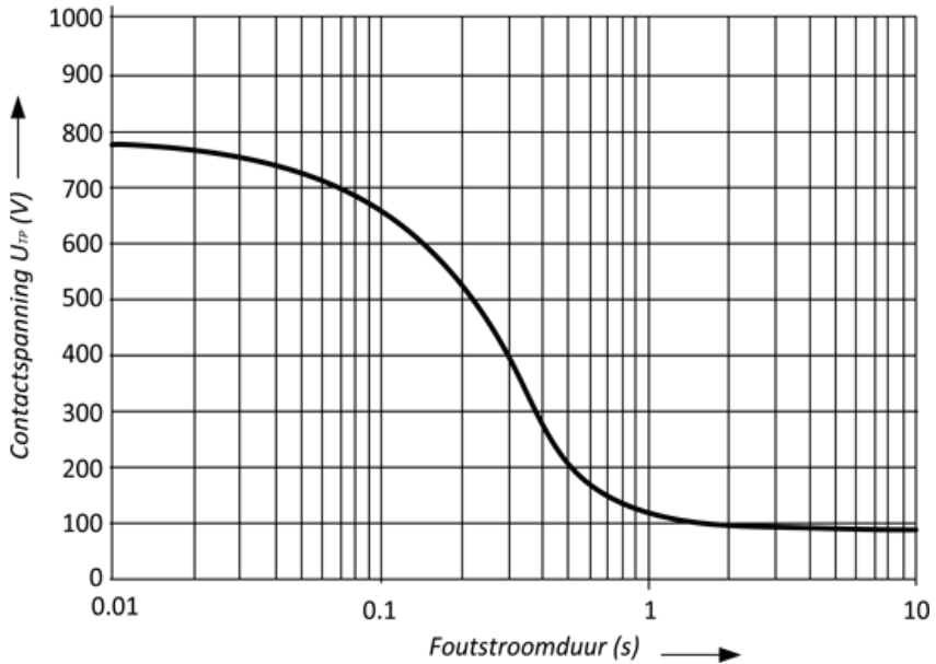
Figuur 2.10. Toelaatbare contactspanning U_{TP} in functie van de foutstroomduur
