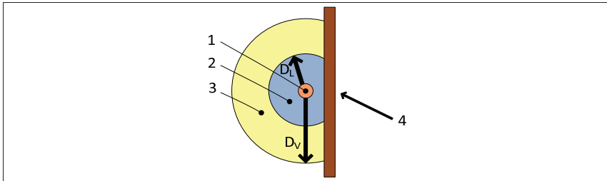
Figuur 2.29. Voorstelling van de zone onder spanning en de nabijheidszone met isolerende bescherminrichting
