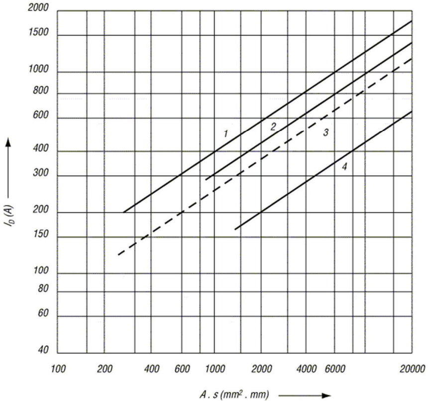
Figuur 5.47. Stroom I_D voor de aardgeleiders met rechthoekige doorsnede in functie van het product van de doorsnede en de omtrek ( A \times s )
