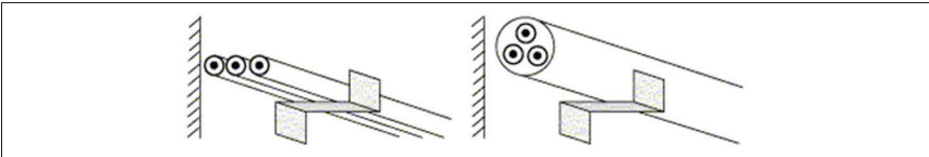
Figuur 5.27. Plaatsingswijzen van elektrische leidingen — Haken
