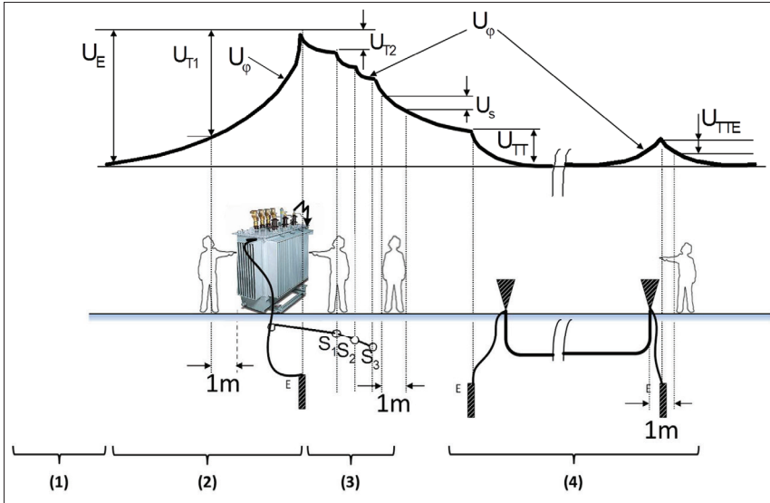
Figuur 2.12. Voorbeeld van verandering van aardbodemspansing en van spanningen bij het vloeien van stroom in de aardverbindingen
