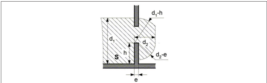
Figuur 2.8. Genaakbaarheidsgabariet: materiële elementen die het verplaatsingsoppervlak begrenzen hebben openingen die geen doorgang verlenen aan een lange staaf van 12 mm diameter
