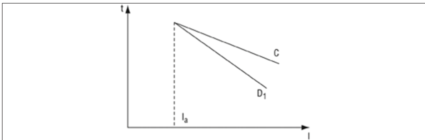
Figuur 5.44. Keuze van de beschermingsinrichting tegen kortsluitingen bij automatische schakelaars (minimale kortsluitstroom)
