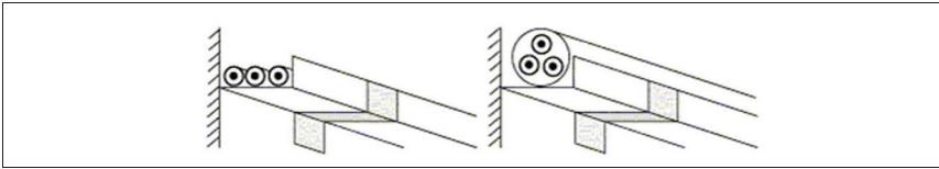
Figuur 5.26. Plaatsingswijzen van elektrische leidingen — Kabelrekken
