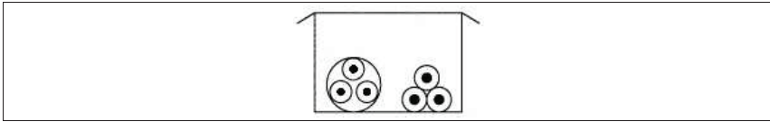
Figuur 5.34. Plaatsingswijzen van elektrische leidingen — Kabelbaan
