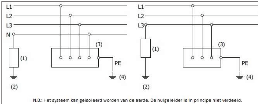
Figuur 2.5. IT-systeem
