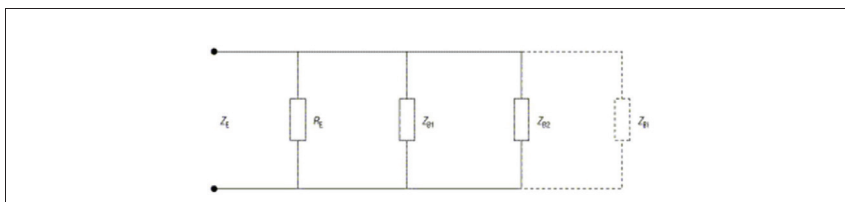
Figuur 2.9. Equivalent schema van de aardingsimpedantie Z_E
