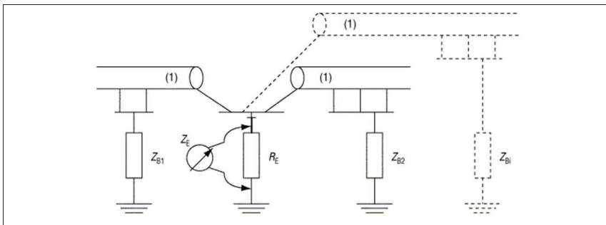
(1) HS-kabel
