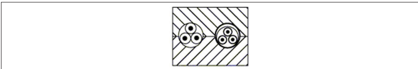
Figuur 5.16. Plaatsingswijzen van elektrische leidingen — Geprefabriceerde blokken
