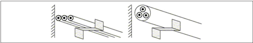
Figuur 5.6. Plaatsingswijzen van elektrische leidingen — Haken
