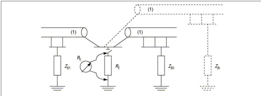
(1) HS-kabel
