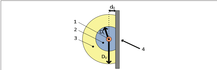
Figuur 2.22. Voorstelling van de zone onder spanning en de nabijheidszone met gearde, metalen bescherming
