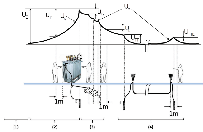
Figuur 2.6. Voorbeeld van verandering van aardbodemschijf en van spanningen bij het vloeien van stroom in de aardverbindingen
