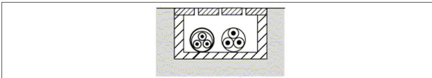
Figuur 5.11. Plaatsingswijzen van elektrische leidingen — Buizen in open of verluchte kabelkanalen
