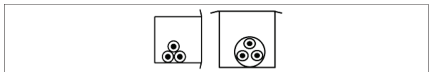
Figuur 2.16. Plaatsingswijze «kabelbaan»
